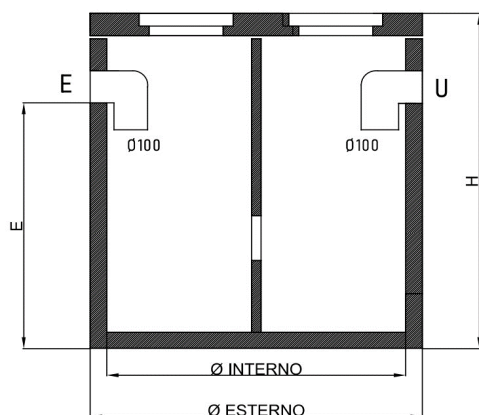
SEZIONE VERTICALE
