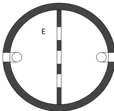
SEZIONE ORIZZONTALE
